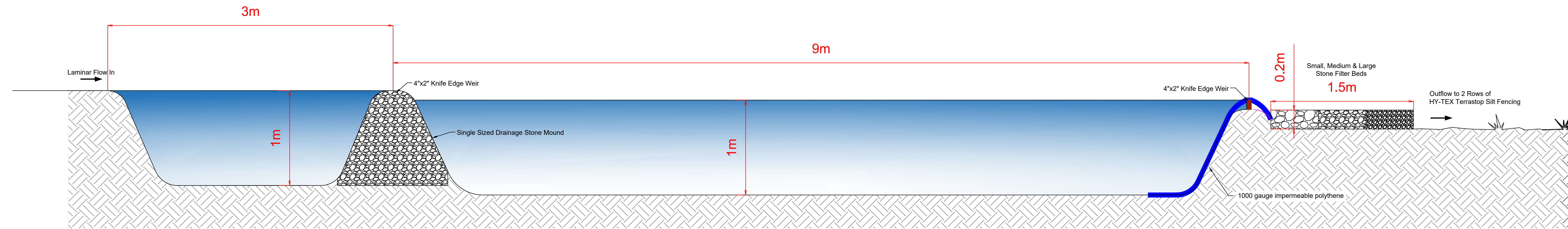
Section A-A
